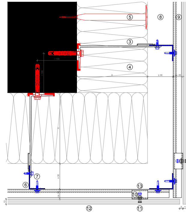
Horizontalschnitt - Aussenecke / horizontal section - external corner
