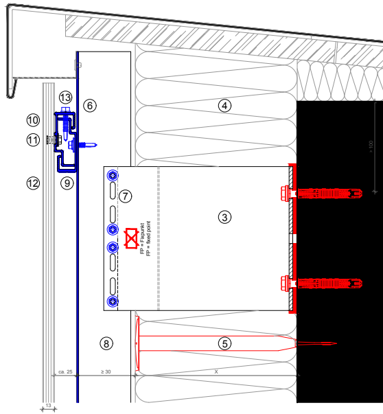
Vertikalschnitt - Dachanschluss Attika / vertical section - head detail
