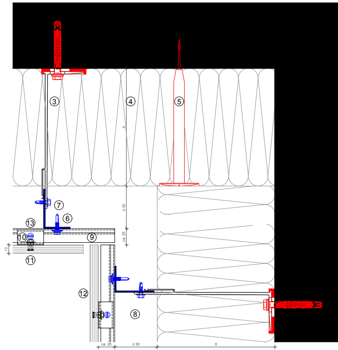
Horizontalschnitt - Innenecke / horizontal section - internal corner
