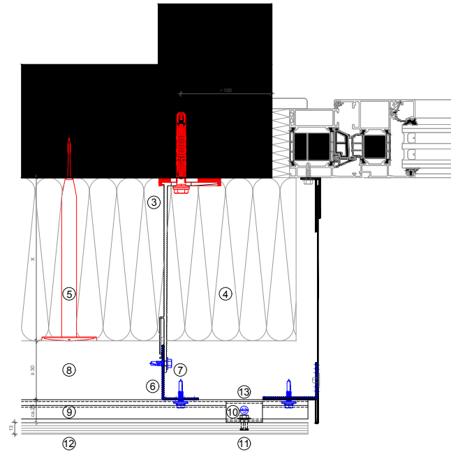
Horizontalschnitt - Fensterleibung / horizontal section - window - reveal
