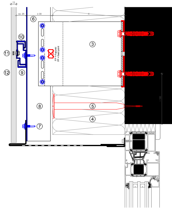
Vertikalschnitt - Fenstersturz / vertical section - window - lintel
